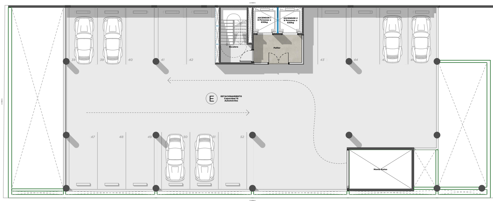
PLANTA DE ENTREPISO
