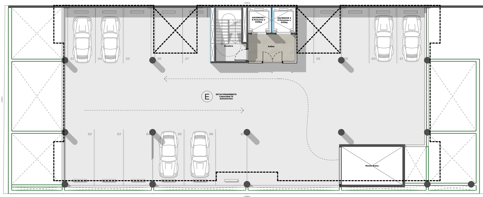
PLANTA DE ENTREPISO 2
